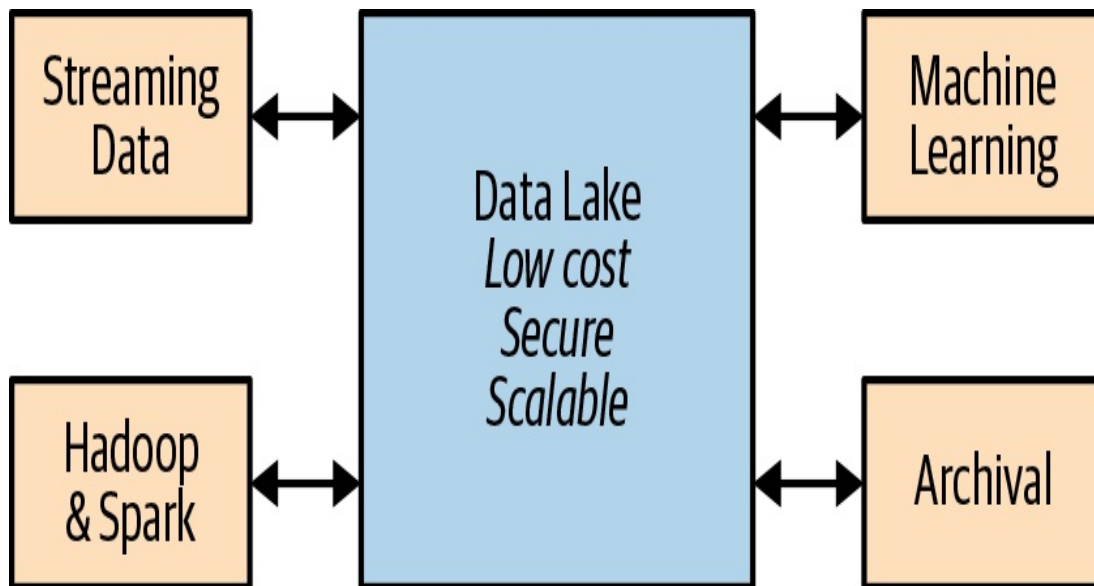
Figure 15-3. Data lake
