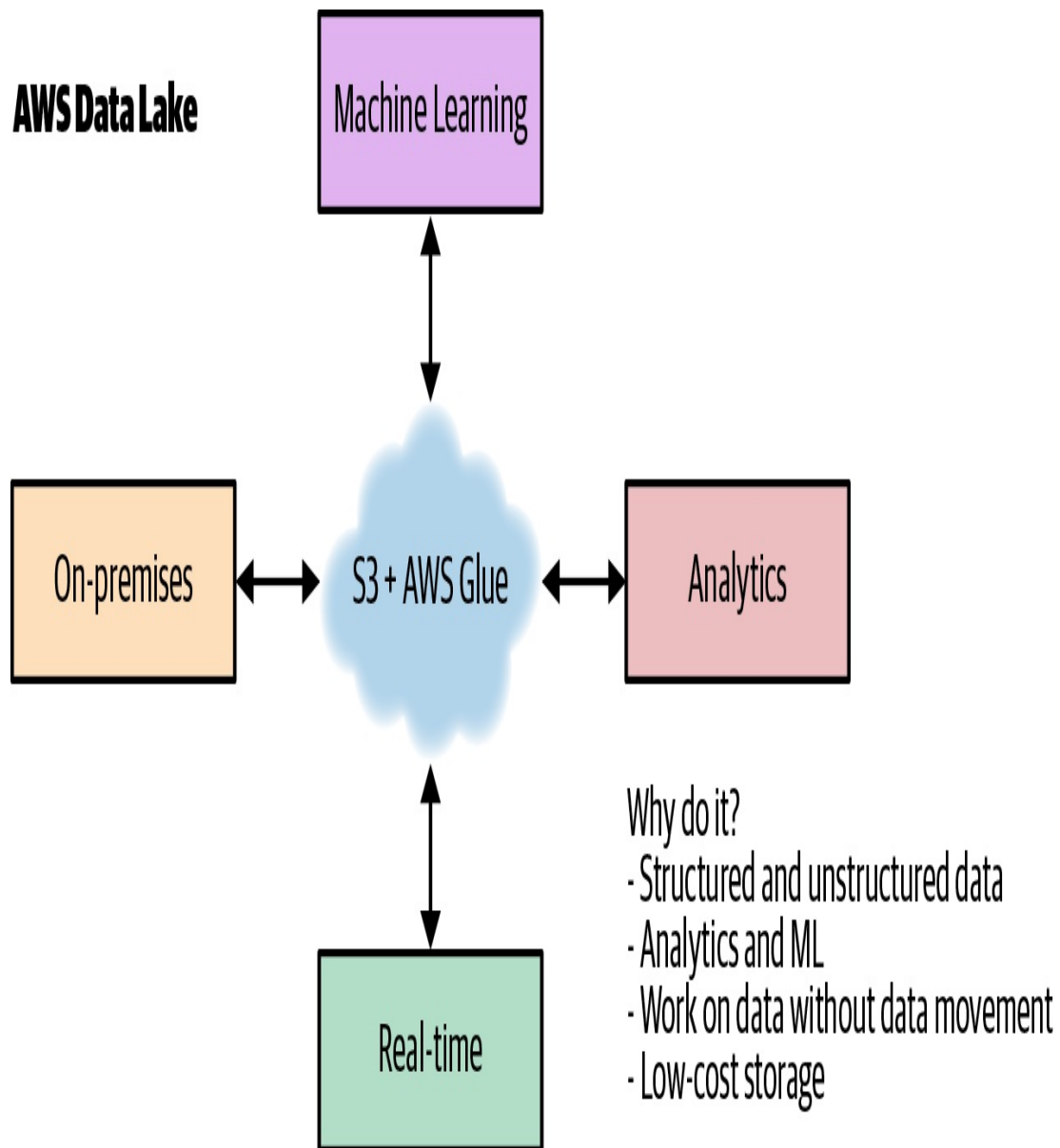
Figure 14-9. AWS data lake
